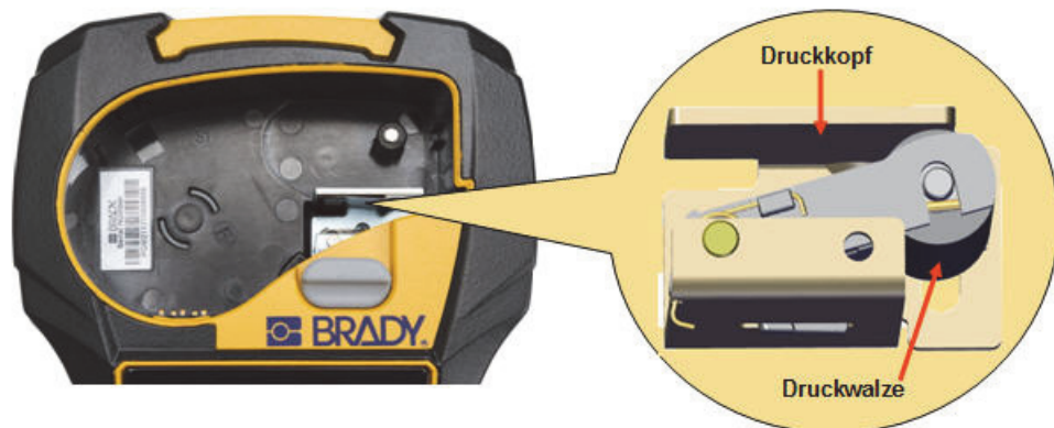
Abbildung 9 • Druckkopf und Druckwalze im Kassettengehäuse
